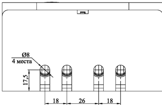
Рисунок А.1 - Размеры счетчика в исполнении D
